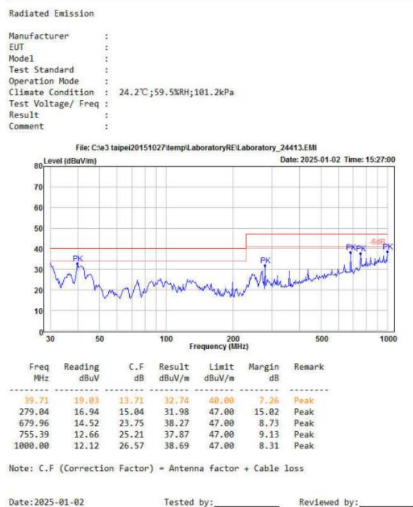
图 4-6 RE 测试垂直方向
